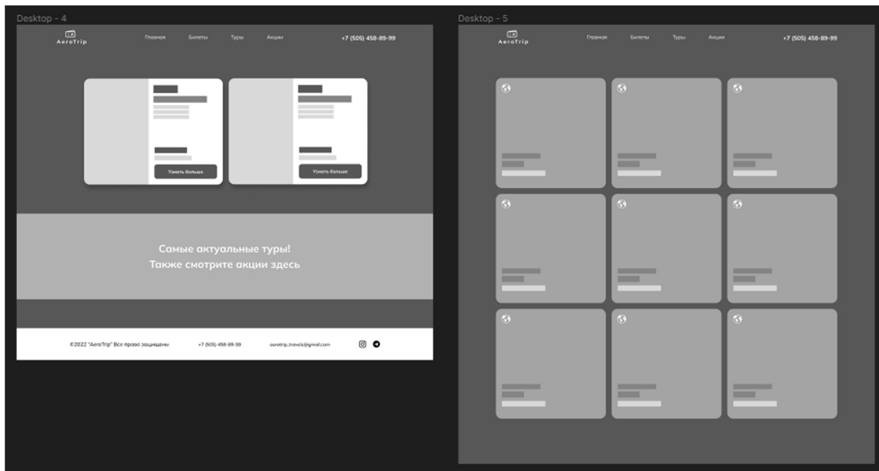
Рисунок 1. Wireframes
